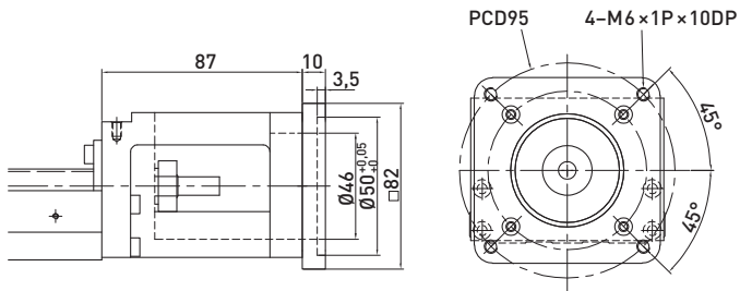
Adapter flange F10
