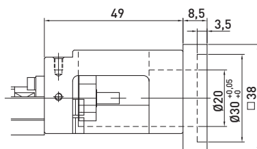
Adapter flange F2
